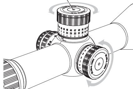
Vis de centre de la molette de hauteur (même design pour la molette de fardage)
