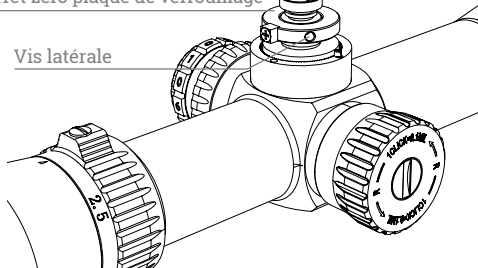
Arrêt zéro plaque de verrouillage
